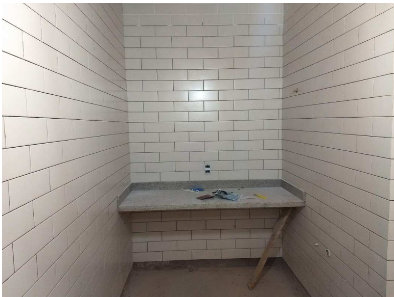
Detalhe do apoio para trocador e da bancada dos banheiros em granito com porta bolsa
