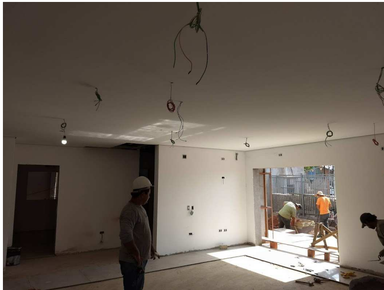
Detalhe da fiação da iluminação da secretaria e da sala de espera
