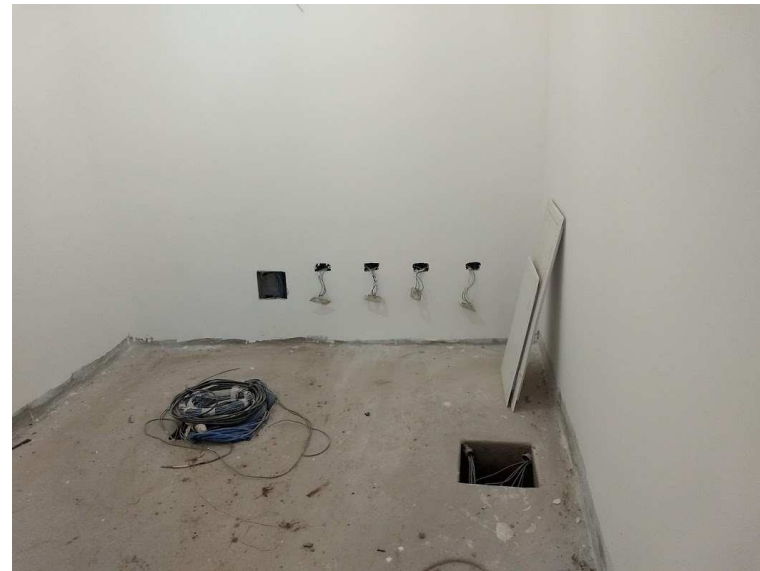
Caixas de passagens sob o piso elevado e detalhe da chegada do cabeamento estruturado na sala técnica
