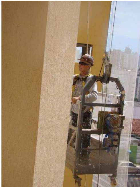
Detalhe do processo de emboço externo com balancim
