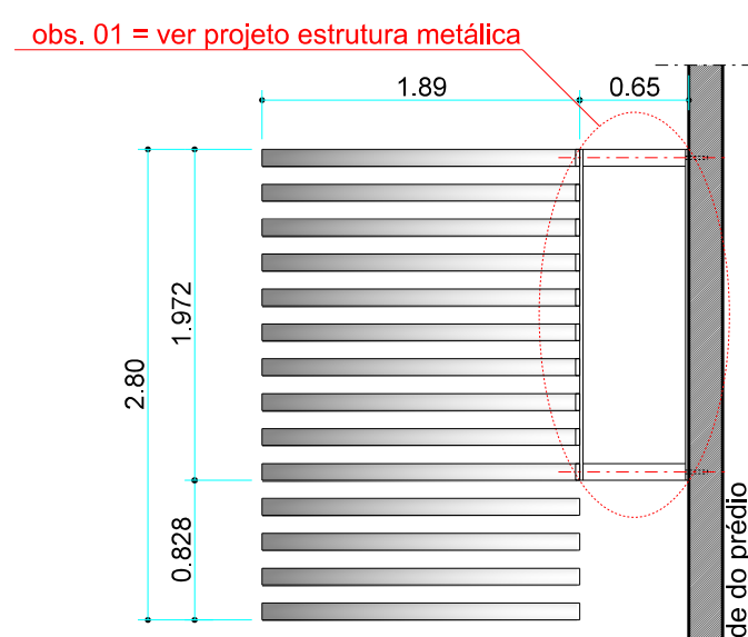
Corte A
