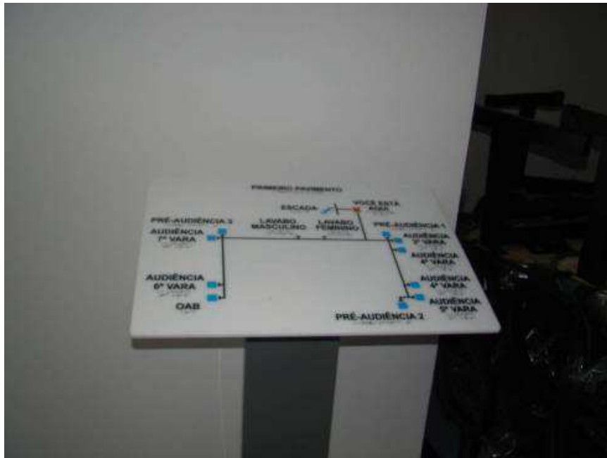
Detalhes Mapa tátil em acrílico com pedestal E Piso tátil PVC alerta e direcional 25x25cm
