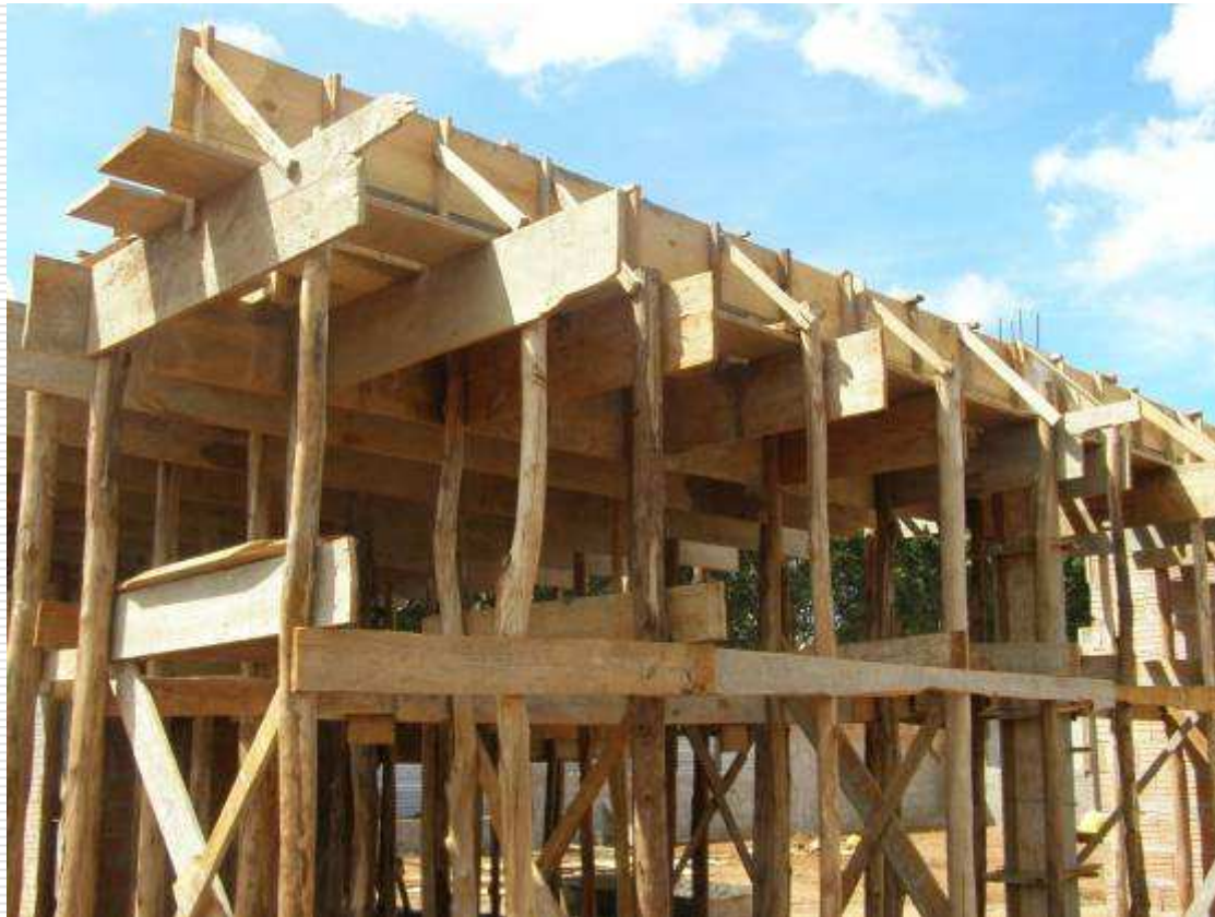
Detalhe da forma da laje em balanço
