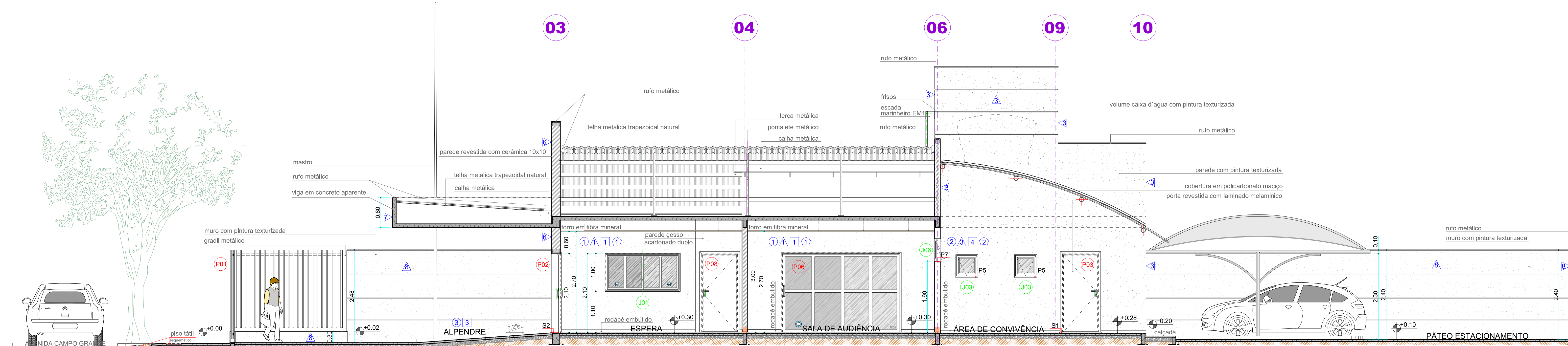
Corte BB
