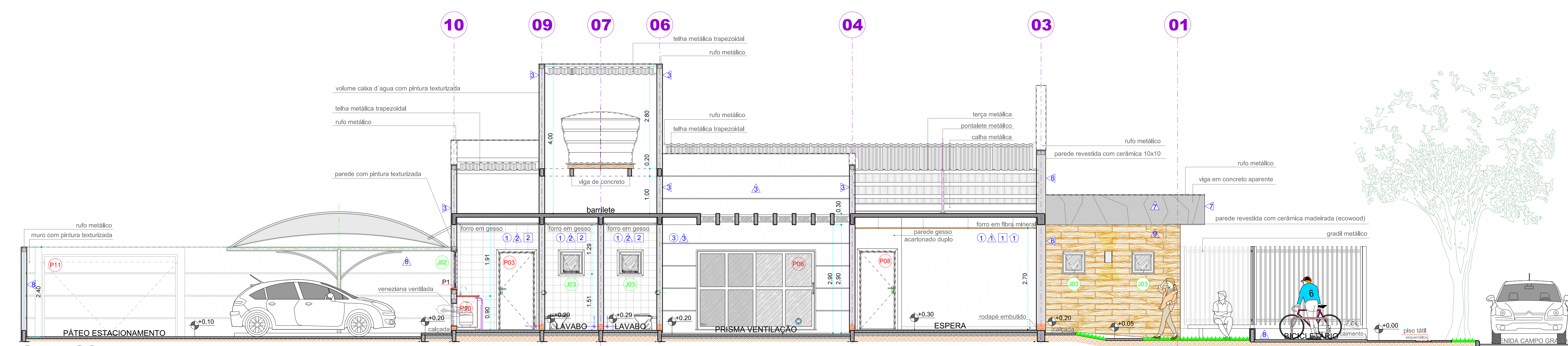
Corte CC
