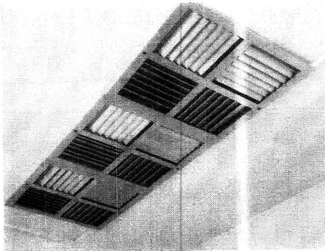
Foto 6 – Rede de dutos- Sala de Extração
