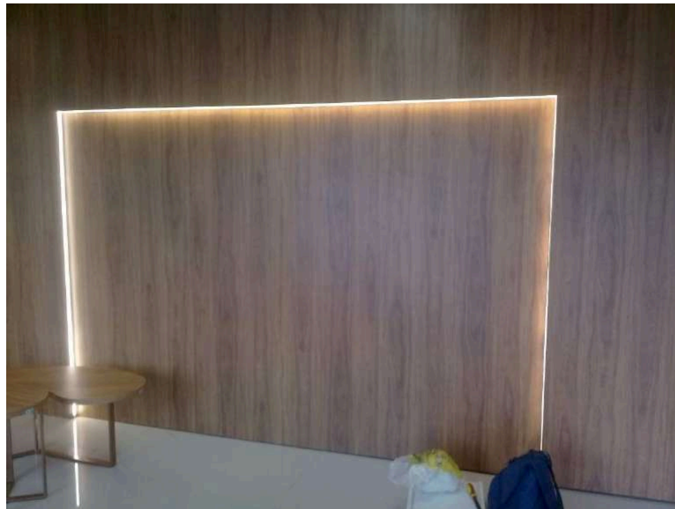
Painel de MDF com laminado Cumaru finalizado e com as fitas de LED
