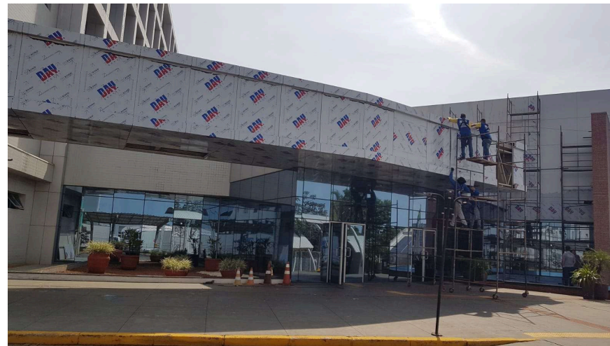
Substituição e instalação do ACM na fachada
